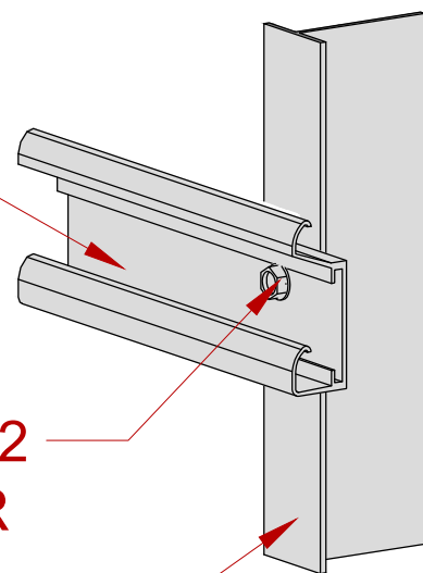
DETALHE FIXAÇÃO VERTICAL - HORIZONTAL
